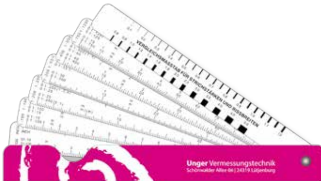
RF 50/3 mit 7 Linealen im Etui aus Aluminiumverbund vernietet. RF 50/3 riveted with 7 rulers in case out of aluminium composite.
